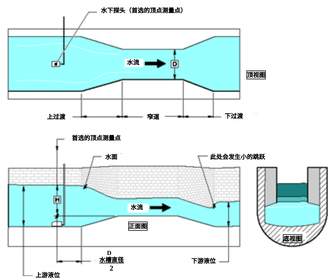
图 53 Leopold-Lagco 型水槽
